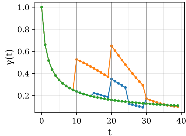
Hartmann-6D
